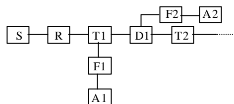
Fig. 3.- Diagrama de un alimentador radial puro.
