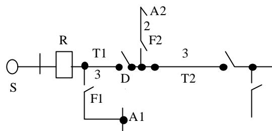
Fig. 2.- Parte de un alimentador radial puro
