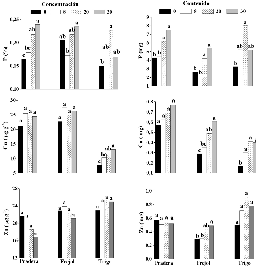
Figura 4: Efecto de la adición de compost en un Ultisol Metrenco, con dosis 0, 8, 20 y 30 Mg ha -1 sobre concentración y contenido de P, Cu y Zn foliar en cultivos de pradera, frejol y trigo sembrados en macetas e incubadas en invernadero. Para cada cultivo barras con la misma letra no difieren estadísticamente, test de Tukey ( \alpha = 0.05 ).
