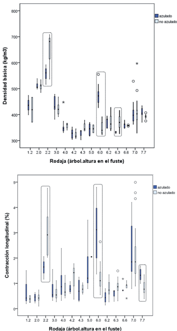
Figura 1. Efecto del azulado en la variación de la densidad básica (arriba) y de la contracción longitudinal (abajo) en la madera de pino silvestre. Las cajas representan la distribución de la muestra con/sin azulado en cada rodaja. El primer dígito del nombre de la rodaja indica el árbol de procedencia y el segundo dígito indica la altura de la rodaja en el fuste en metros. Aparecen marcadas las cajas entre las que se hallaron diferencias significativas.
