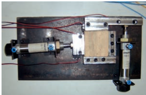
Figura 6. Sistema de sujeción del material.
