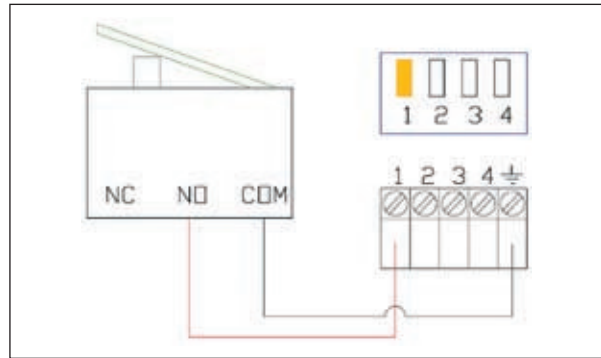
Figura 9. Conexión del microswitch al controlador.
