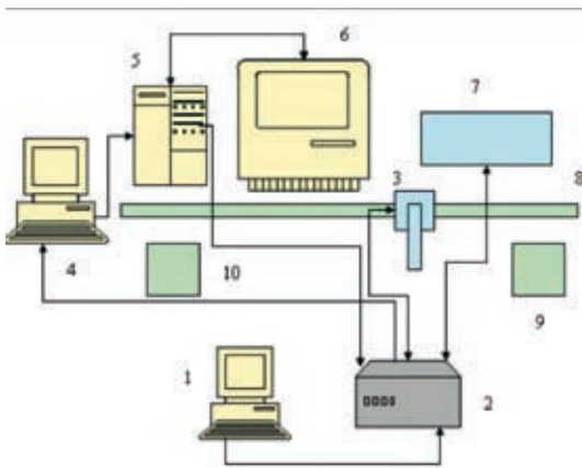
Figura 4. Configuración de la célula de mecanizado.
