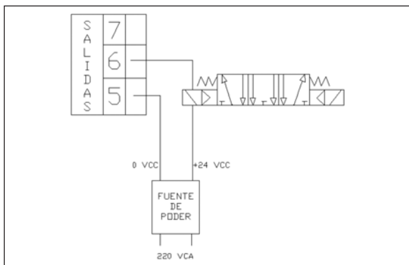
Figura 12. Conexión con las salidas del controlador.
