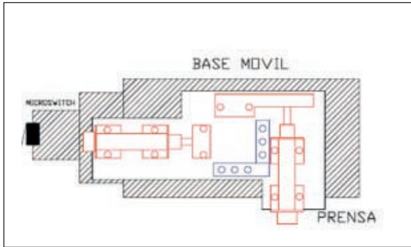
Figura 8. Posición del microswitch.
