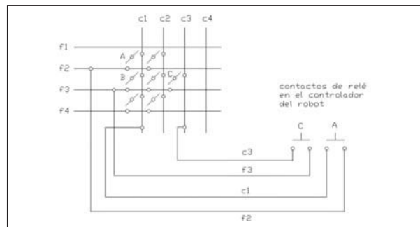
Figura 11. Esquema de conexión interna.
