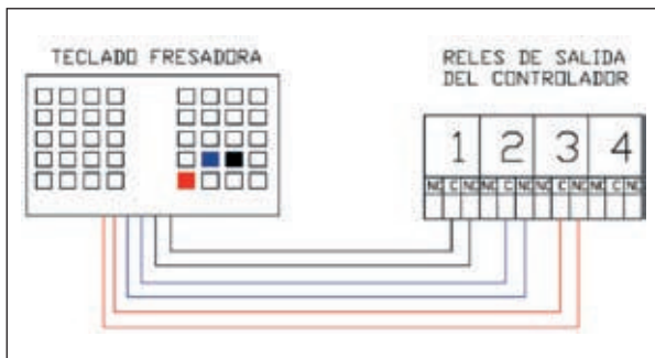
Figura 10. Conexión de las líneas con el controlador.
