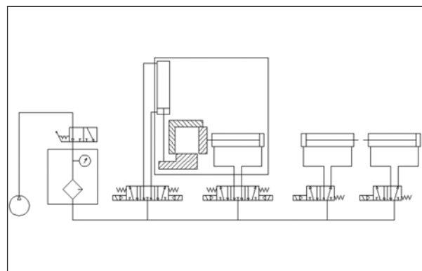
Figura 13. Esquema del circuito electroneumático.
