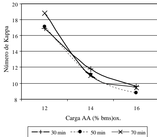
Figura 3. Efecto de la carga de álcali activo y tiempo a T máx sobre el número de Kappa.
