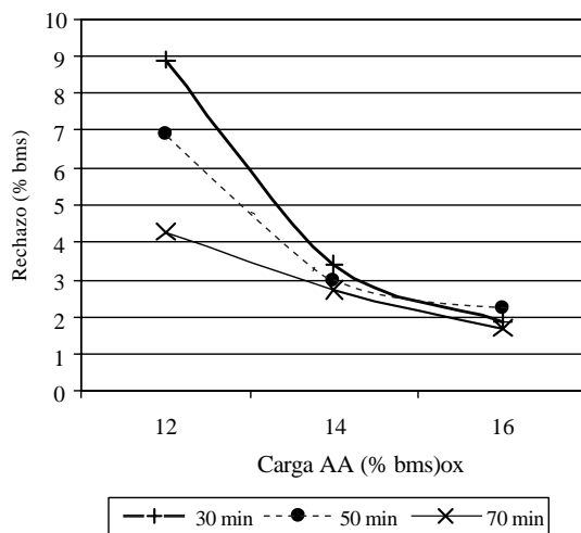
Figura 2. Efecto de la carga de álcali activo y tiempo a T máx sobre la obtención de rechazo.
