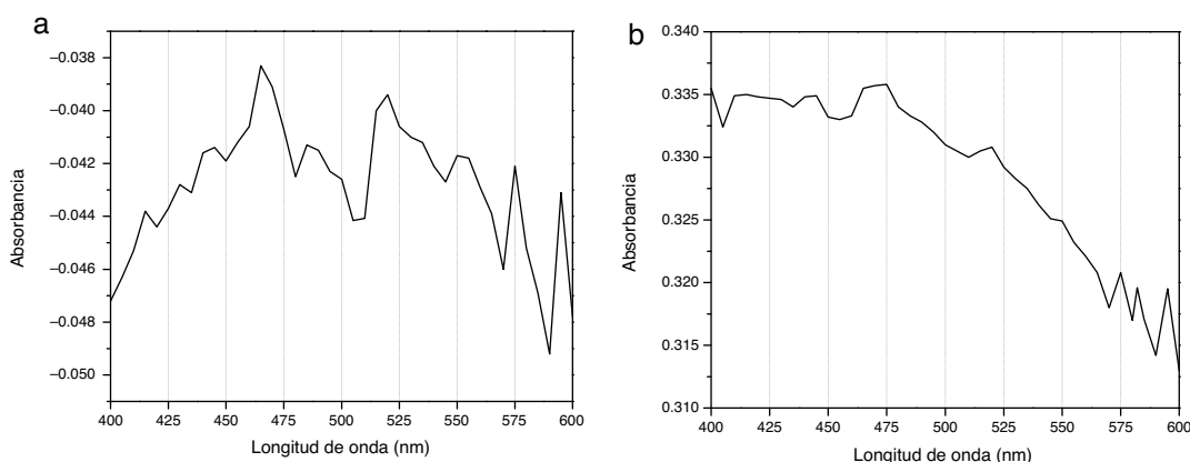
Figura 5 El espectrograma «a» corresponde al espectro de absorción de CHX al 2% no tratada y el espectrograma «b» corresponde al espectro de absorción de CHX al 2% activada con ultrasonido endodóntico por 90 seg.
