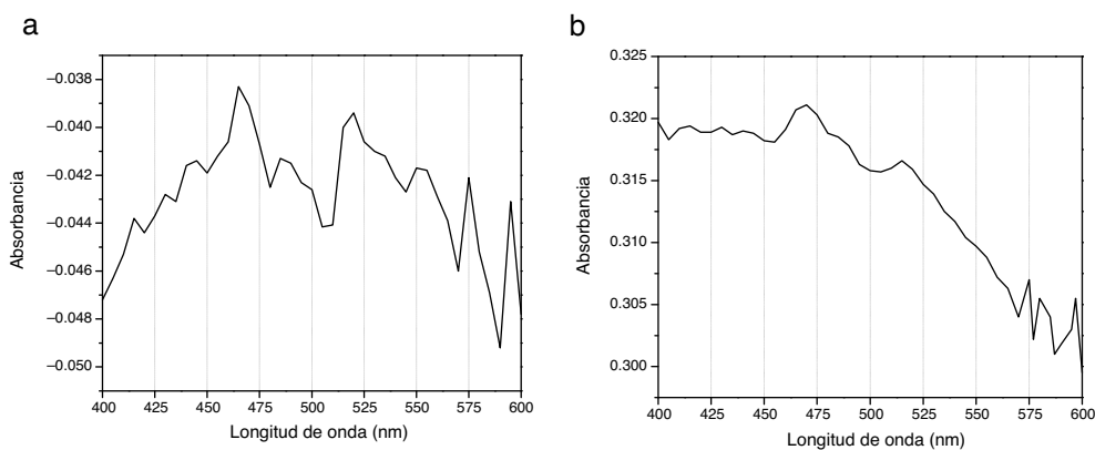
Figura 6 El espectrograma «a» corresponde al espectro de absorción de CHX al 2% no tratada y el espectrograma «b» corresponde al espectro de absorción de CHX al 2% activada con ultrasonido endodóntico por 120 segundos.
