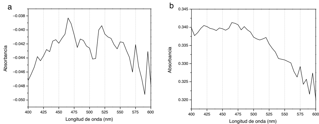
Figura 4 El espectrograma «a» corresponde al espectro de absorción de CHX al 2% no tratada y el espectrograma «b» corresponde al espectro de absorción de CHX al 2% activada con ultrasonido endodóntico por 60 seg.
