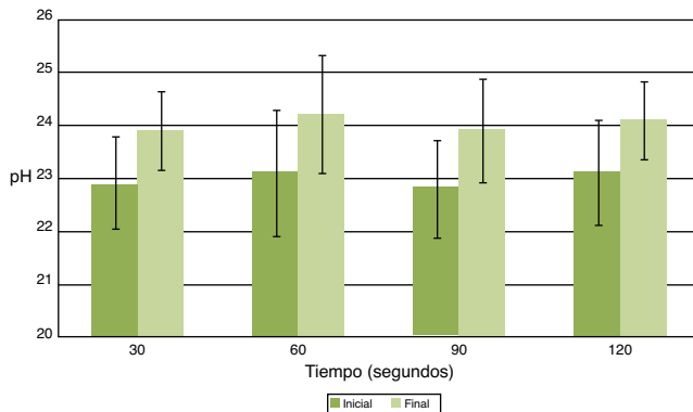
Figura 2 Valores promedio de temperatura y desviación estándar para clorhexidina 2% sometida a ultrasonido endodóntico (USE) a una frecuencia de 24.500 Hertz. Las diferencias entre el antes y el después para todos los tiempos de aplicación de USE no son significativas.
