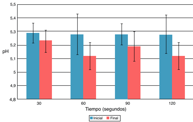
Figura 1 Valores promedio de pH y desviación estándar para clorhexidina 2% sometida a ultrasonido endodóntico (USE) a una frecuencia de 24.500 Hertz. Las diferencias entre el antes y el después para todos los tiempos de aplicación de USE no son significativas.
